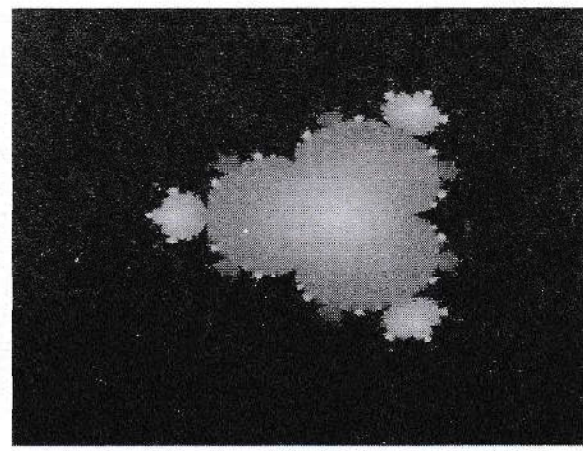
Fig. 15. G. F. f(z) = z^4 + c , c = -.6 + 0i
