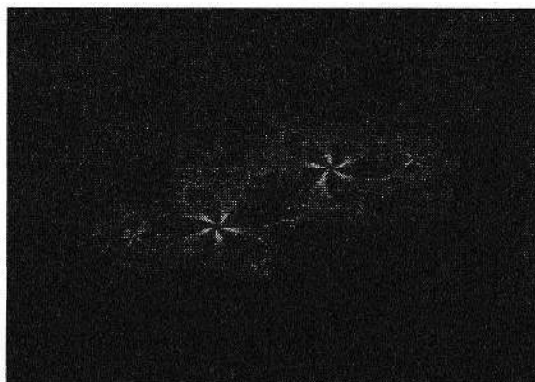
Fig. 2. Julia Set
